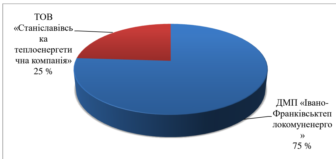
Рис. 2.2.1. Структура розподілу приєднаного теплового навантаження централізованої системи тепlopостачання між тепlopостачальними організаціями
