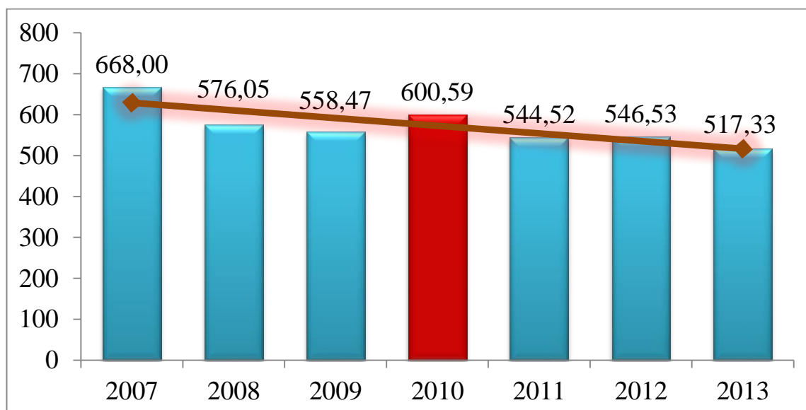
Рис. 2.3.3.Динаміка споживання теплової енергії у м. Івано – Франківську упродовж 2007-2013 рр. , тис. МВт*год
